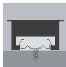
installazione standard a scomparsa
