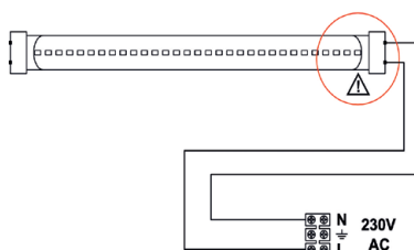
Connessione diretta alimentandi i piedini dalla parte dell'etichetta
